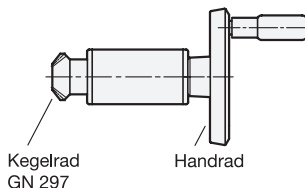
Übertragungseinheit
