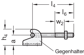
Form TT Zuganker mit T-Stück
