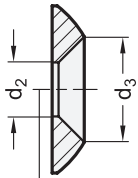
Bore for countersunk head screw DIN 7991 / DIN ISO 2009
