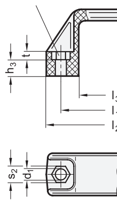
GN 528.3 Bore for hex head screw DIN 931/ISO 4014
