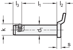
Bolzen-Ø 8 Kugelraste einseitig
