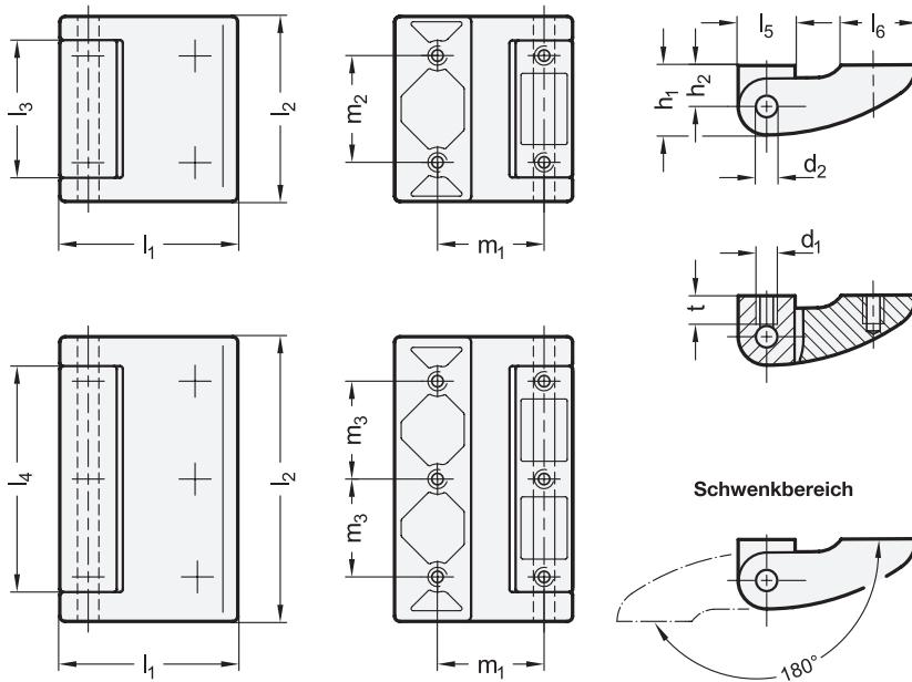
4 Form A Befestigung von der Rückseite
