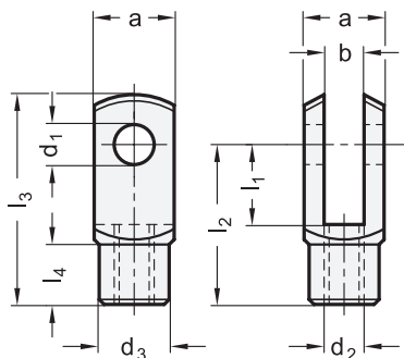
Gabelkopf DIN 71752
