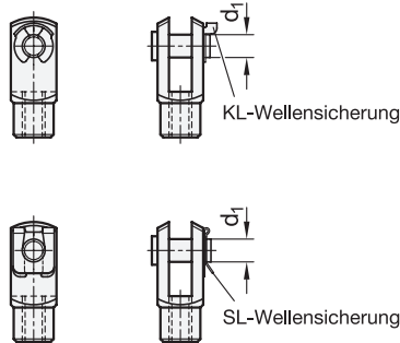
Gabelgelenke GN 751
