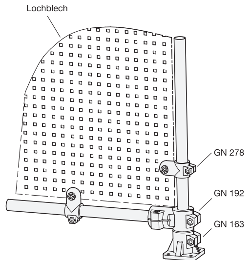
Schutzzaun
